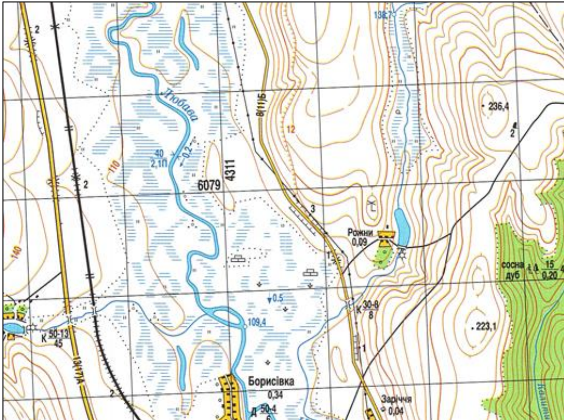
Рисунок Ж.16 – Варіант 1 вихідних даних для визначення по карті витрати води річки Любава
