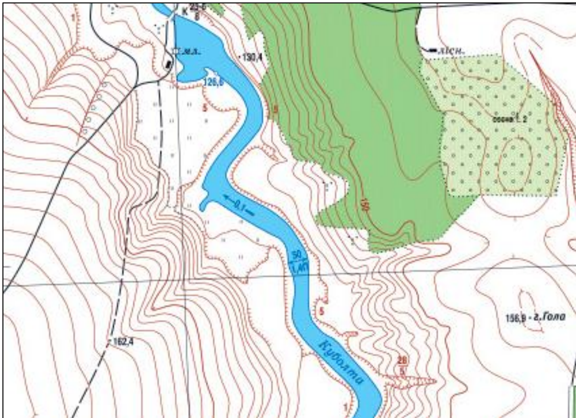
Рисунок Ж.19 – Варіант 4 вихідних даних для визначення по карті витрати води річки Куболта
