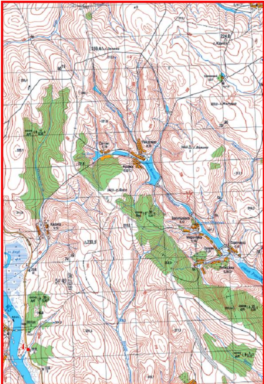
Рисунок Ж.8 – Варіант 3 вихідних даних для визначення і виділення на карті меж водозбірної площі водотоку ( 1 – точка, до якої буде стікати вода з водозбірної площі)
