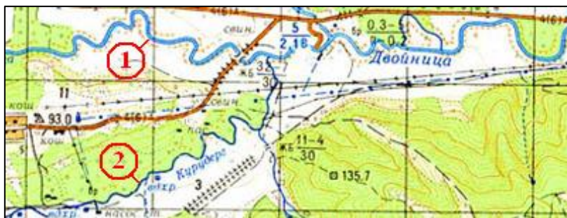
Рисунок 6.2 – Фрагмент топографічної карти, на якій за допомогою лінійних знаків подаються дороги, лінії електропередач, водотоки: 1 – річки шириною від 5 м до 30 м; 2 – річки та струмки шириною до 5 м (зображення з сайту http://www.geoguide.com.ua )
